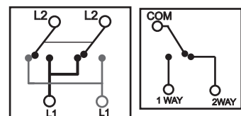
Moduł wyłącznika krzyżowego
